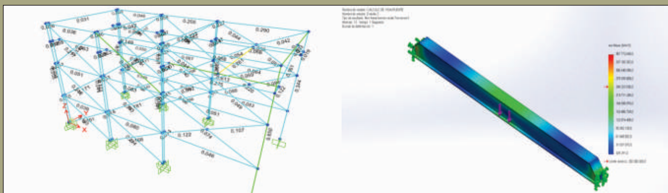
CALCULO ESTRUCTURAL NAVE INDUSTRIAL
